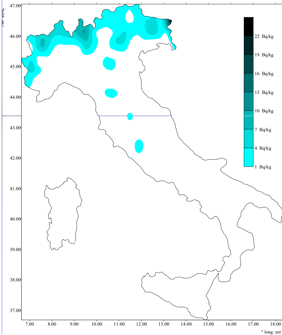
Distribuzione della concentrazione di Cs 137 nei mieli italiani (smelatura '96)
