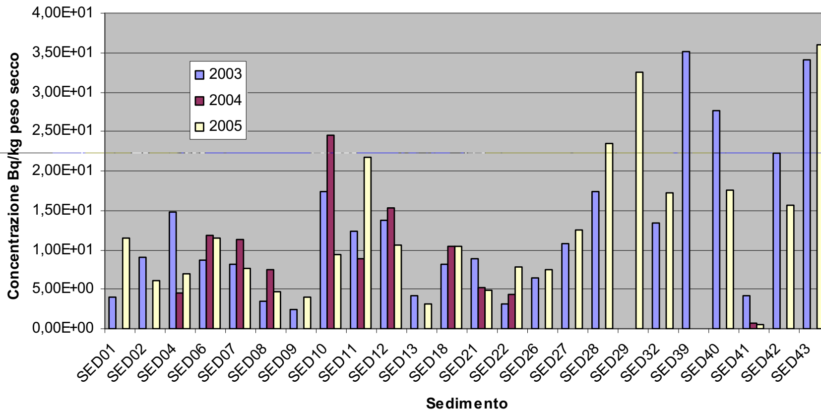
Cs-137 nei sedimenti analizzati
