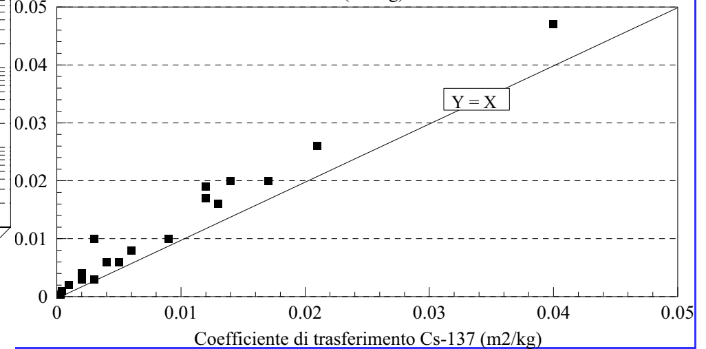
Coefficiente di trasferimento Cs-134 (m 2 /kg)
