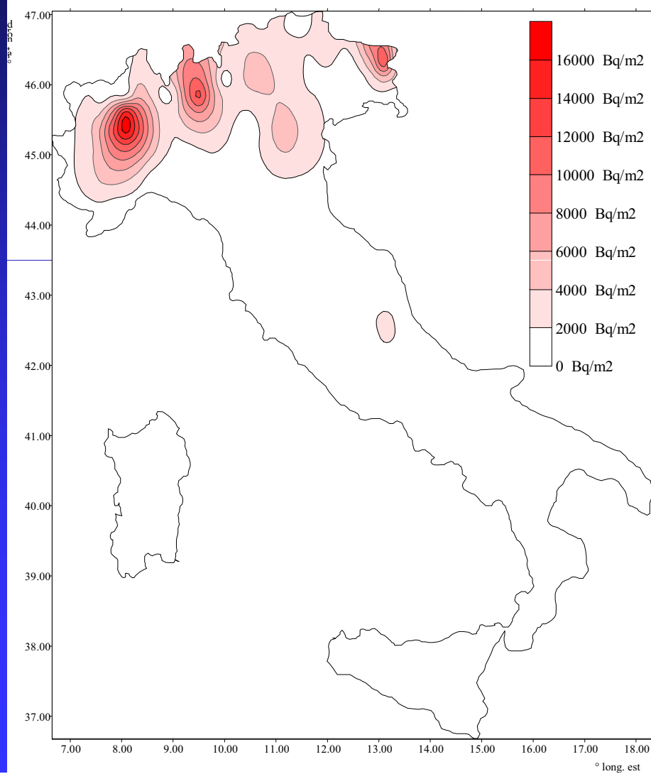
Distribuzione della concentrazione di Cs 137 (Bq/m 2 ) nei muschi della campagna nazionale
