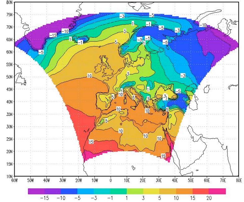
T2m RegCM4 (deg C) JF 1989
