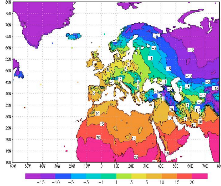
T2m CRU (deg C) JF 1989
