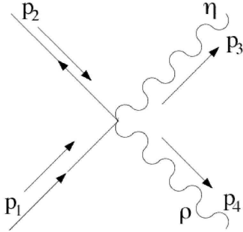
FIG. 14: vertex4
