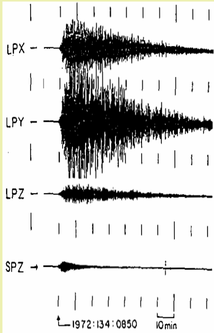
lunar seismograms
